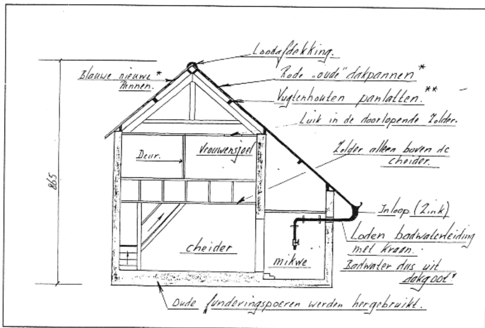
afb.7. Reconstructie dwarsdoorsnede Berghse synagoge 1871 (J. Hoogakker)
