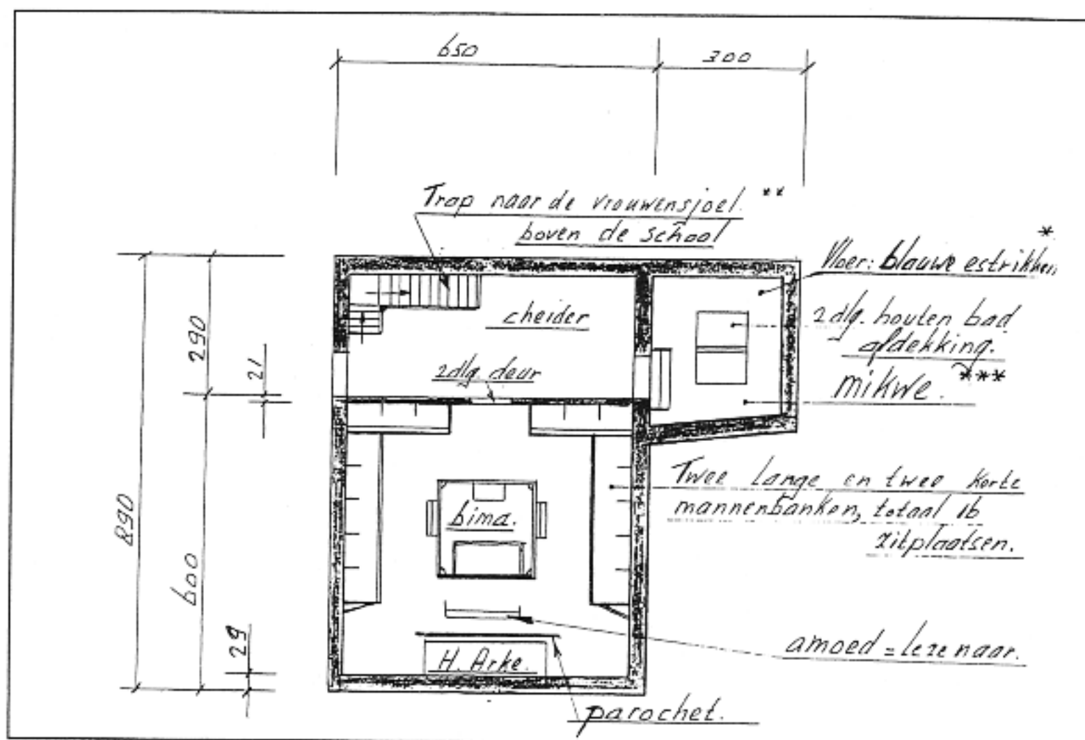
afb.8. Reconstructie grondplan Berghse synagoge 1871 (J. Hoogakker)
