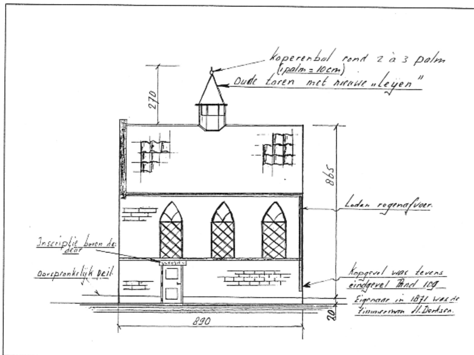
afb.6. Reconstructie Zijgevel "Oost" Berghse synagoge 1871 (J. Hoogakker)
